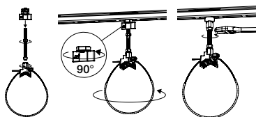
Montáž
