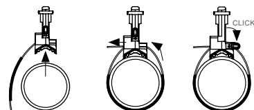
Montáž
